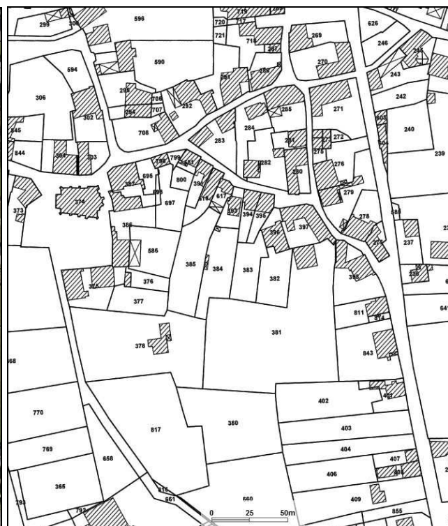
Parcelles cadastrales
